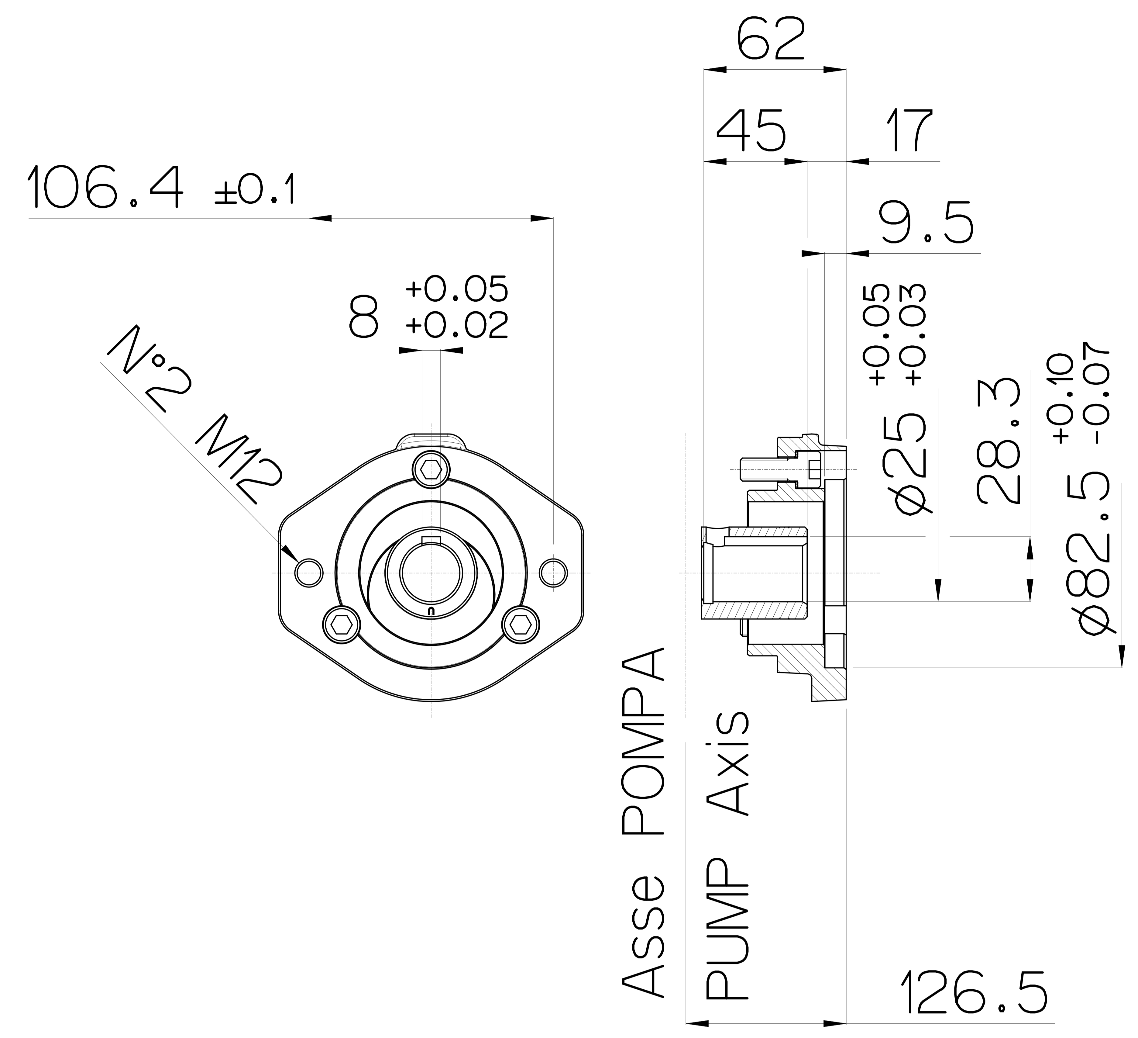
ZETA 350 MI 25 cod. 819800
